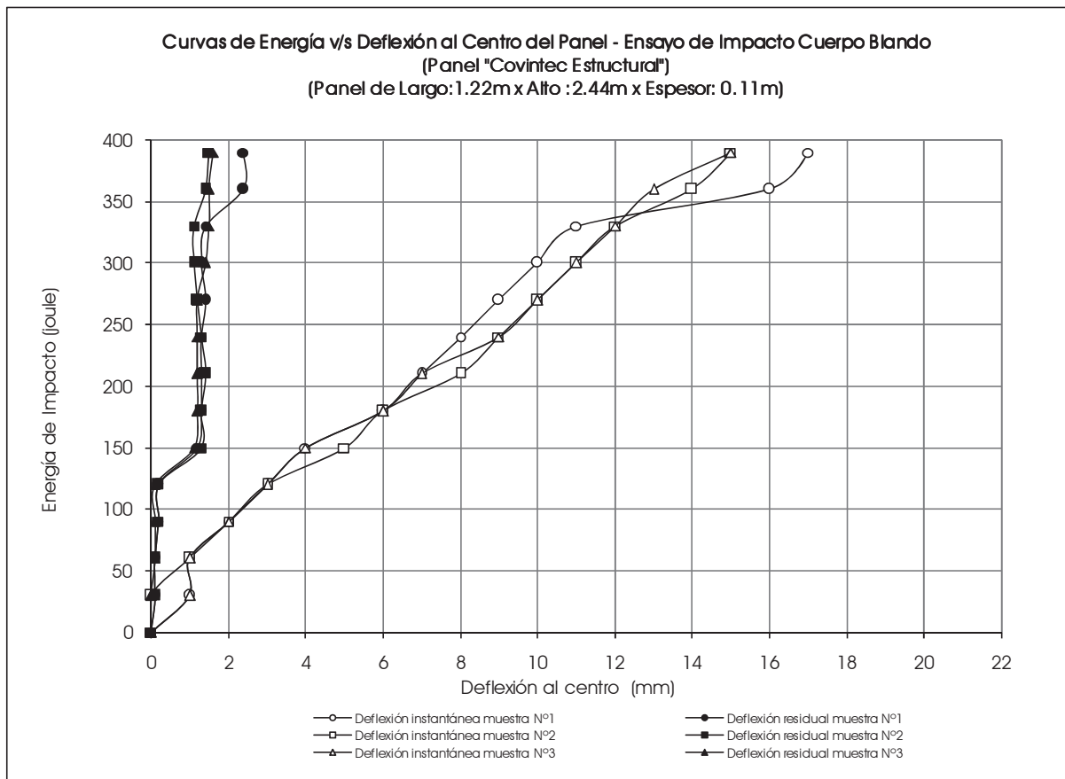
Gráfico 1. Curvas energía de impacto – deformación fuera de plano del panel.
