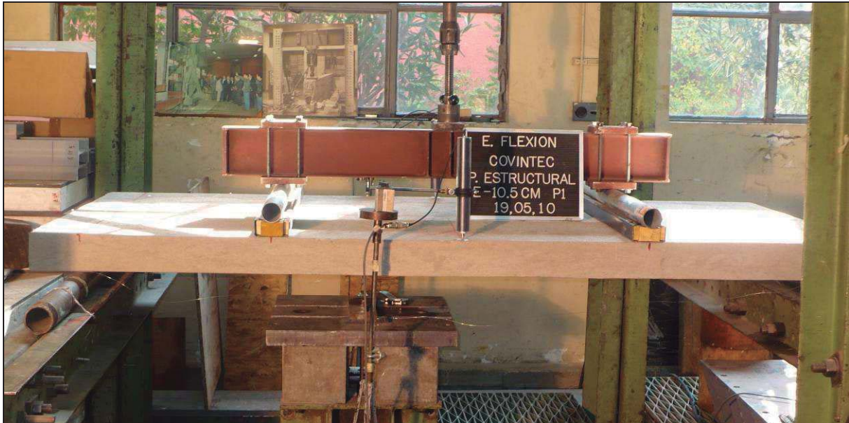
Foto 1. Vista general del montaje del ensayo de flexión al panel.
