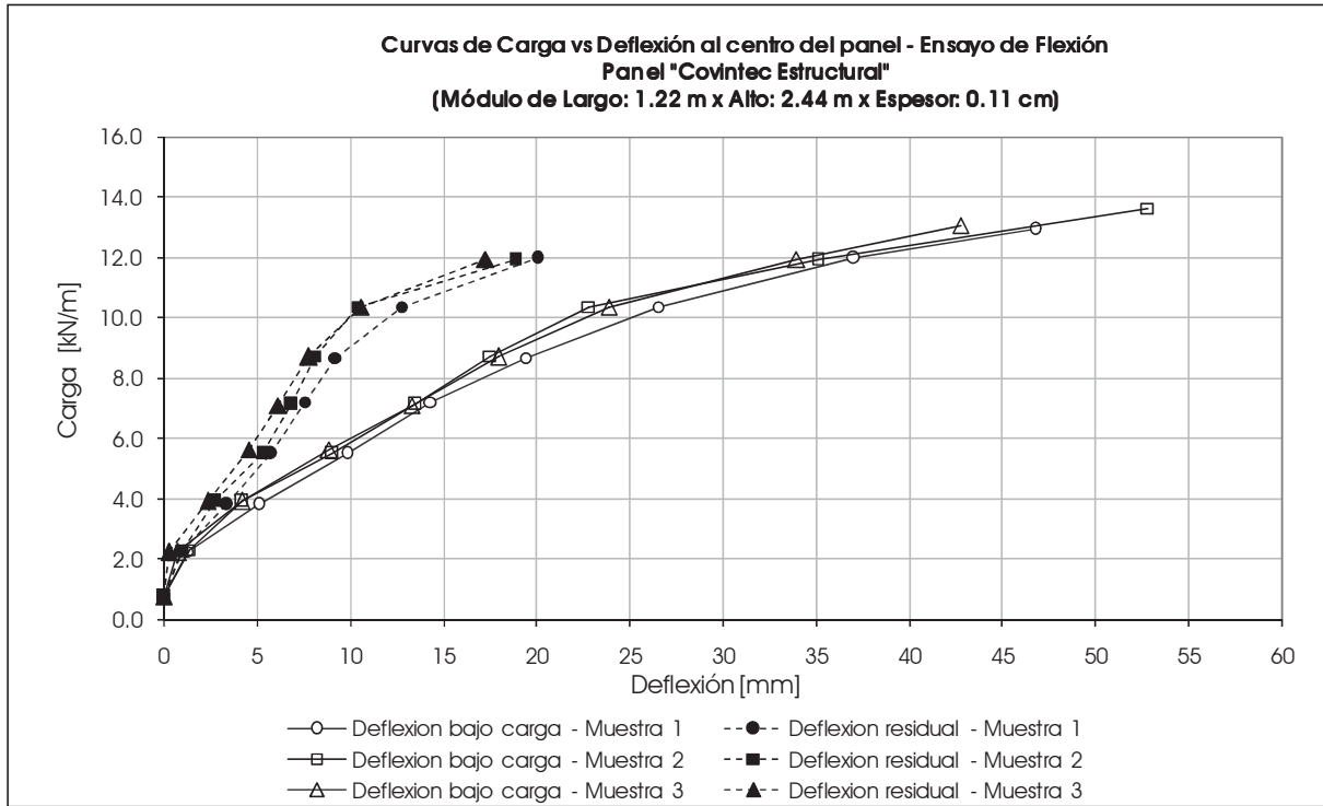
Gráfico 1. Curvas carga – deflexión (carga normalizada por el largo del panel).
